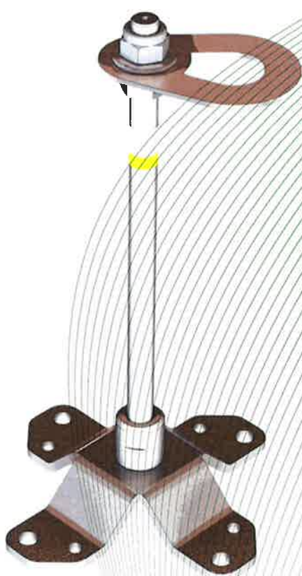
Bild 2: Anschlageinrichtung, Typ: P U4 SP16 mit EAP F
