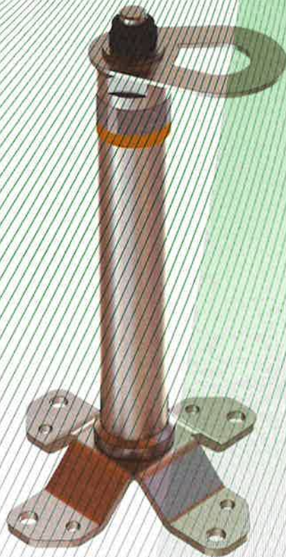
Bild 3: Anschlageinrichtung, Typ: P U4 STR42 mit EAP F
